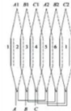
菱形绕组杯平面图
