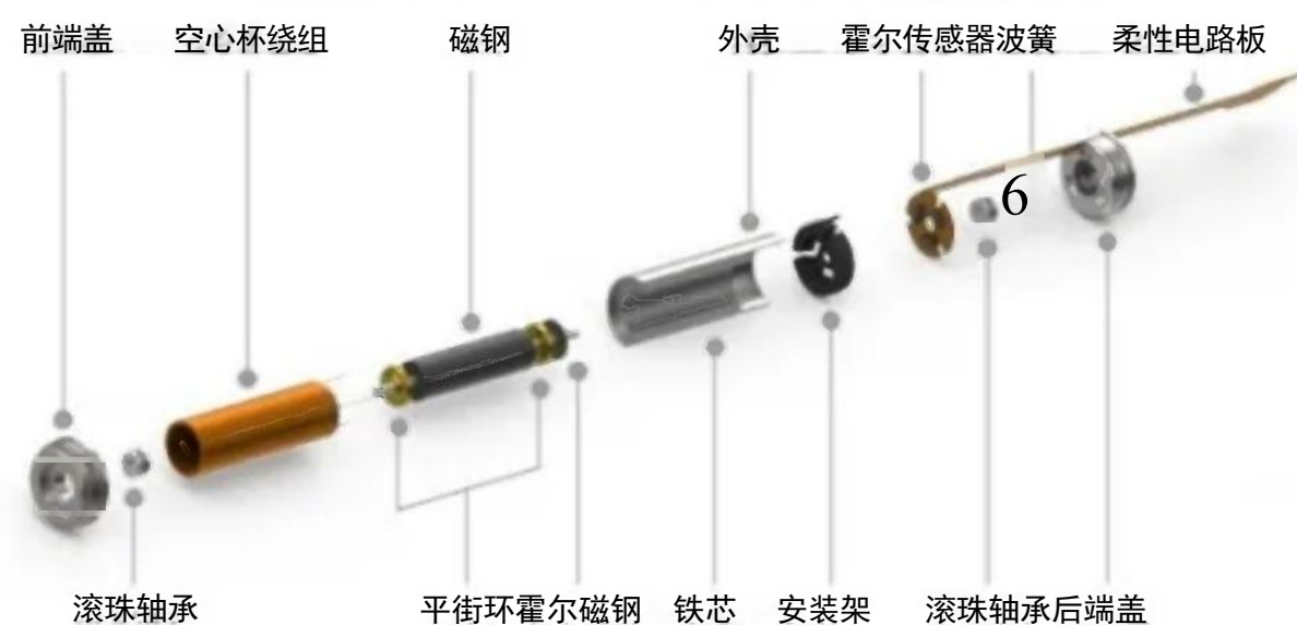
鸣志电器的无刷空心杯电机结构图
