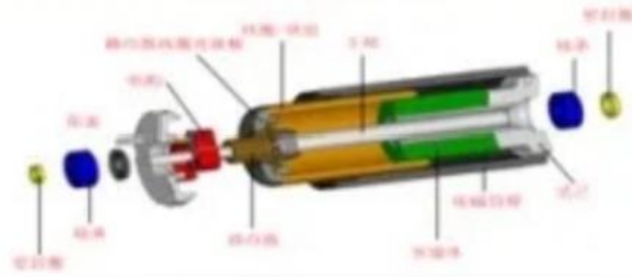
空心杯电机
