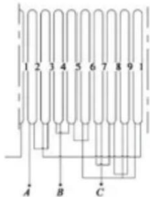
直绕式绕线杯平面连接图
