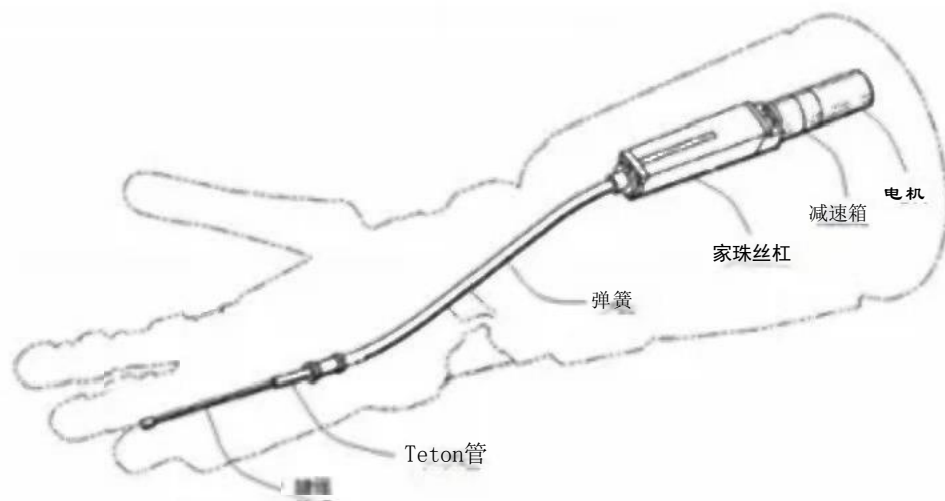
腱驱动原理
