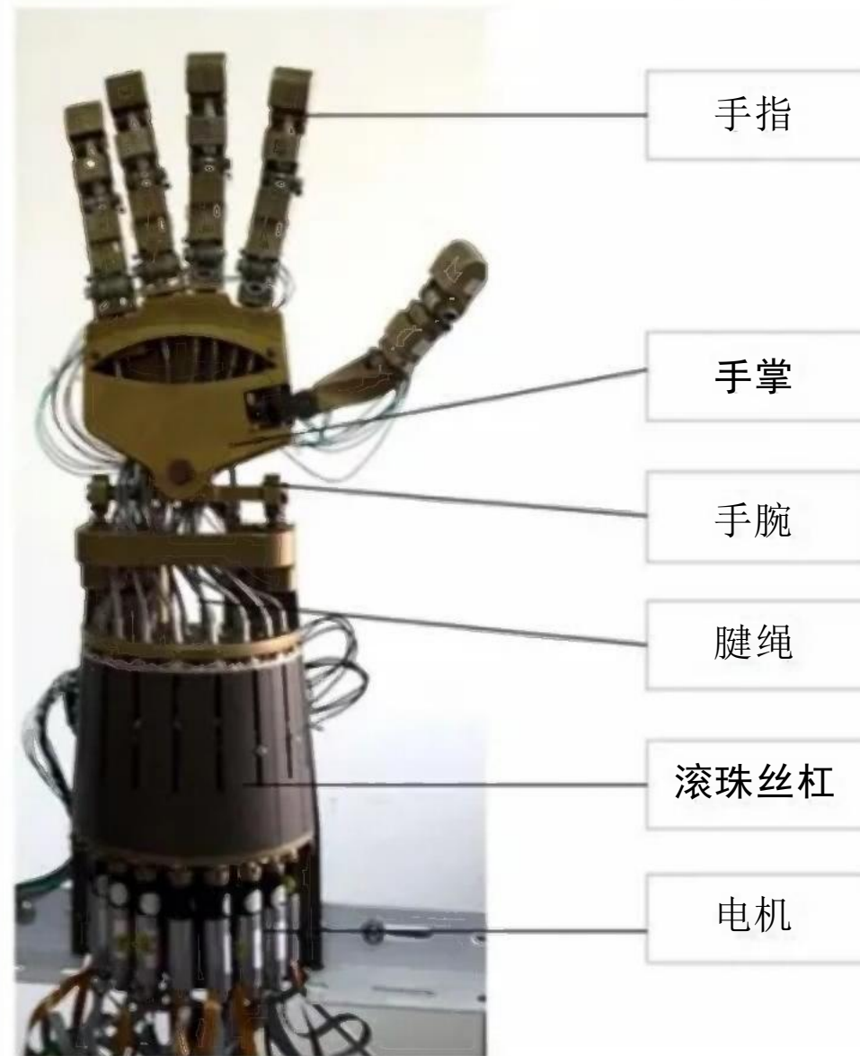
驱动器外置灵巧手整机机构
