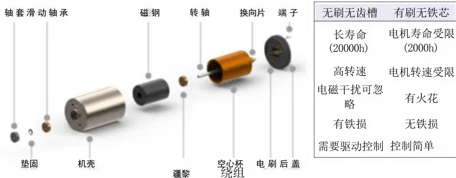
鸣志电器的有刷空心杯电机结构图
